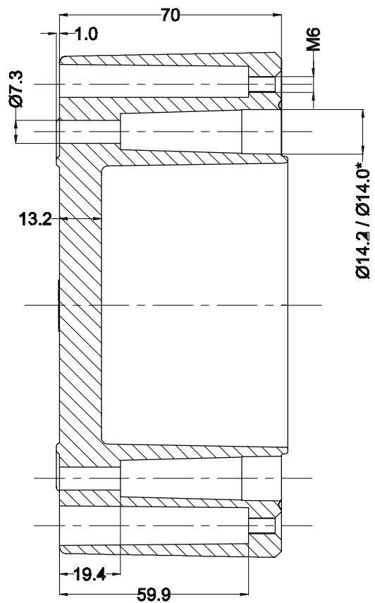
SECTION D-D
