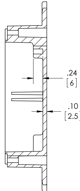
SECTION A-A
