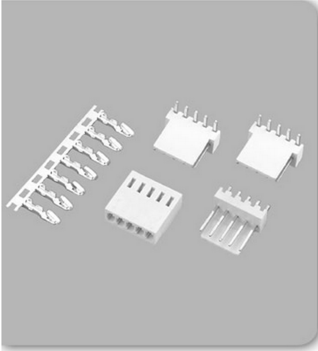
2510-nY 母头
