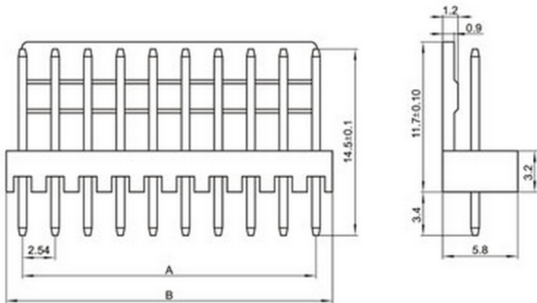
2510-nA 针座
