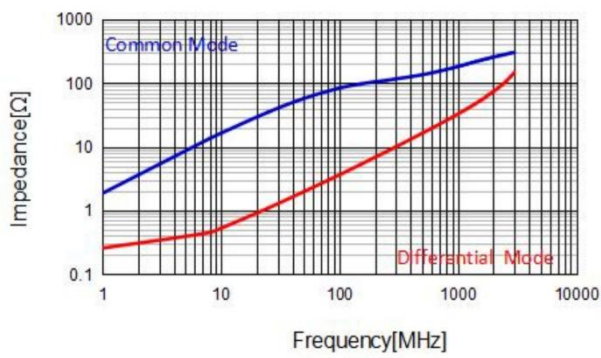
APCW2012-181P2T
