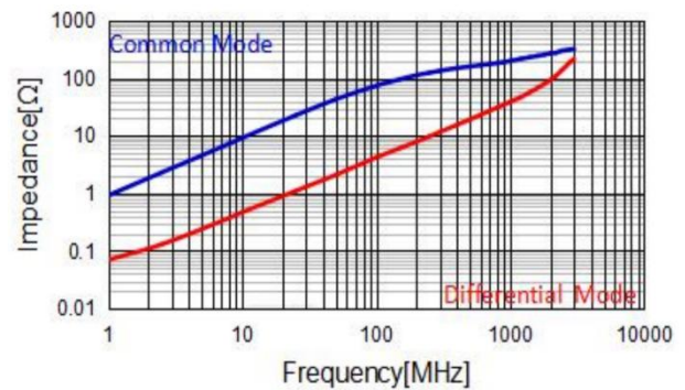
APCW2012-121P2T
