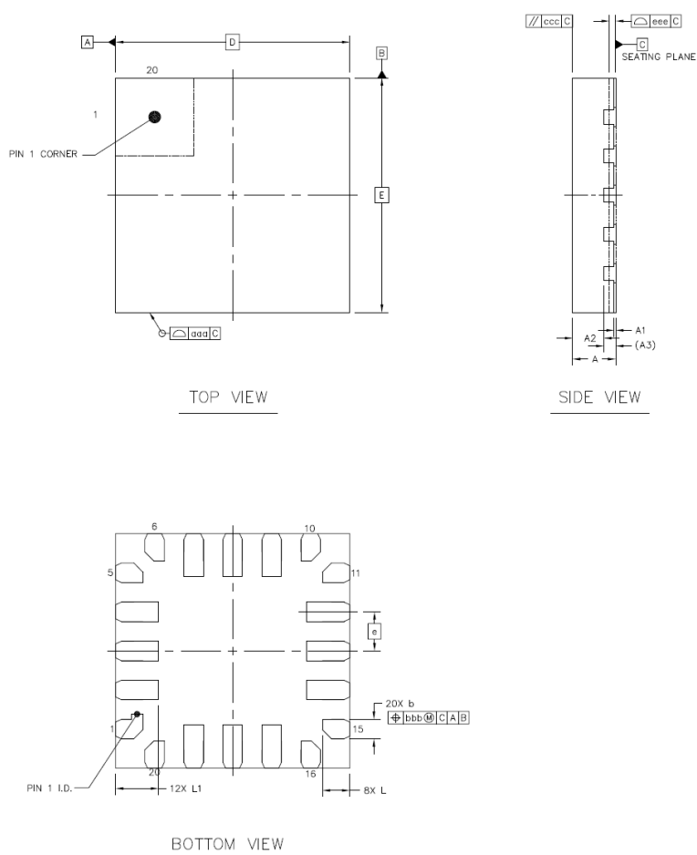
图14 QFN20 封装图
