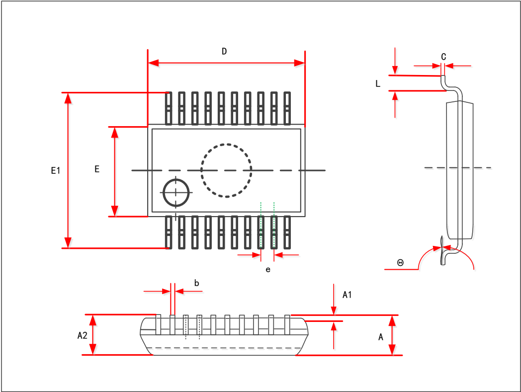
图13 SOP20 封装图
