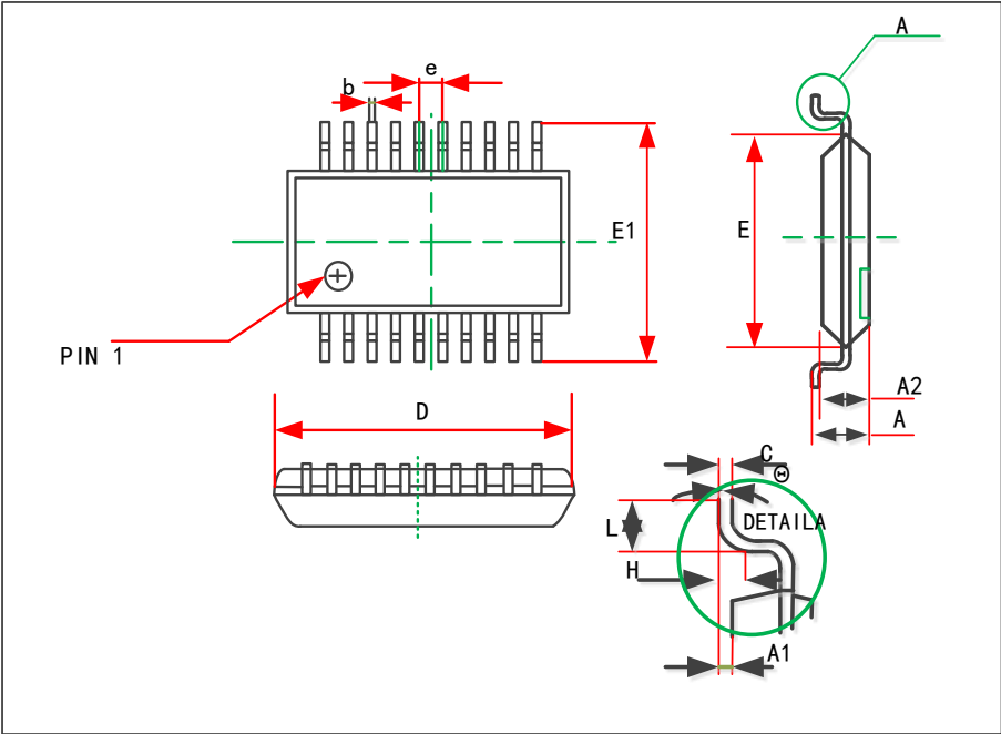
图12 TSS0P20 封装图
