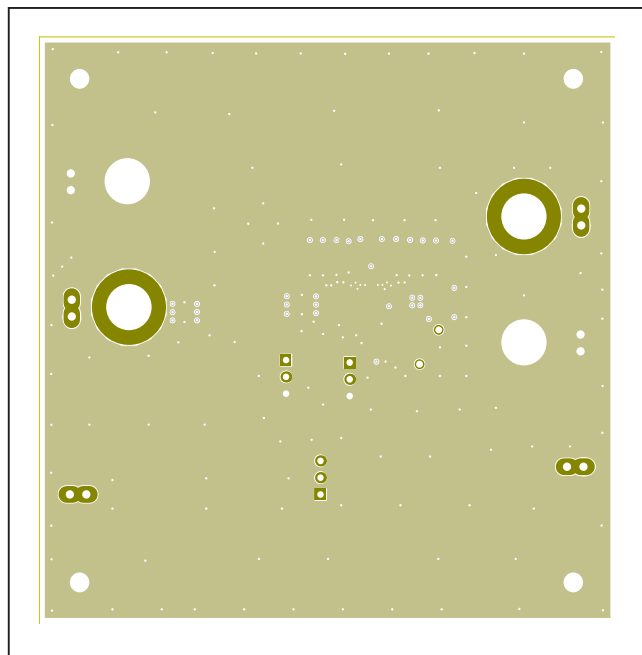
MAX20006E/MAX20008E EV Kit PCB Layout - Internal Layer 2
