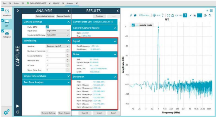
Figure 28. FFT Tab
