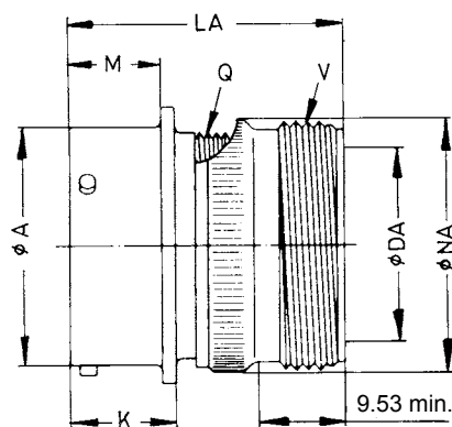
PT 00 A PT 00 C
