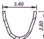
剖面 B-B 比例 5:1
