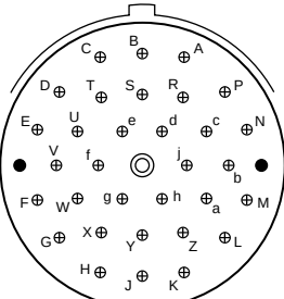
25-32
