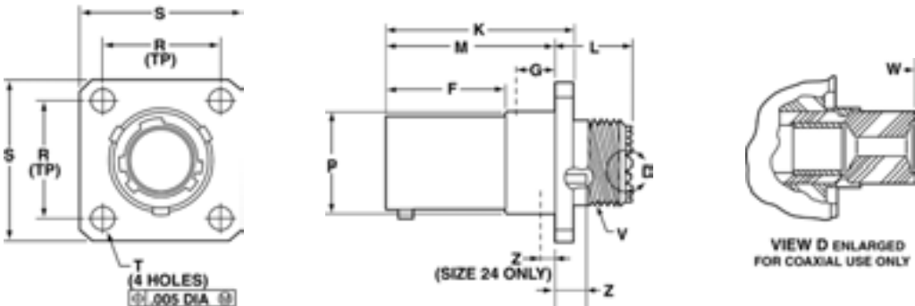
SJTP00RT
