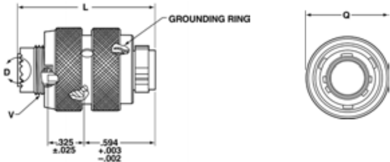
SJTG06RT
