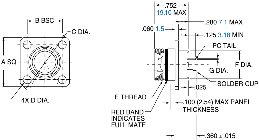
2M801-012-02
