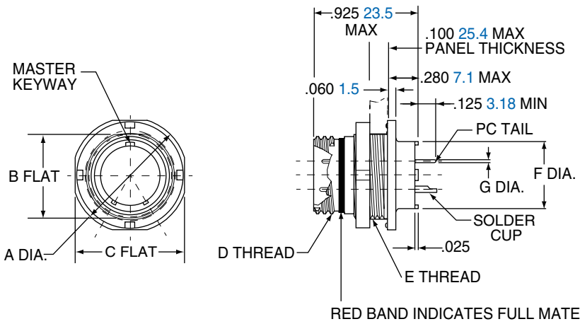
2M801-012-07
