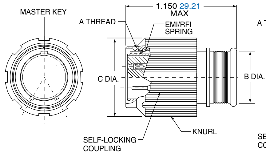
2M805-001
