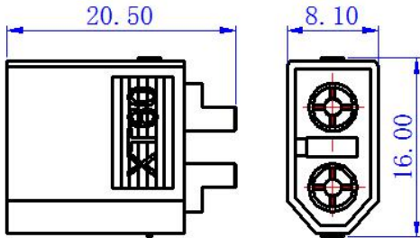
XT60-M
