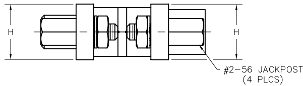
RECEPTACLE
