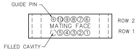
RECEPTACLE MA-221-010-261-A63WA
