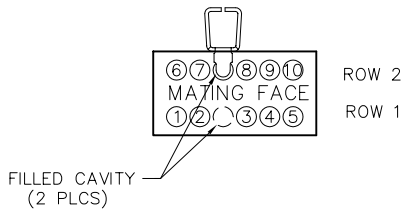
PLUG MA-231-010-161-ABCWA
