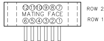
RECEPTACLE MA-281-012-435-A0000
