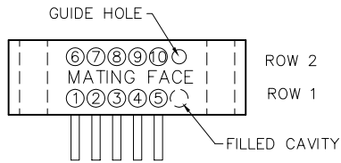
PLUG MA-251-010-325-A6600
