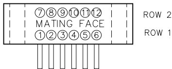
PLUG MA-271-012-325-A0000
