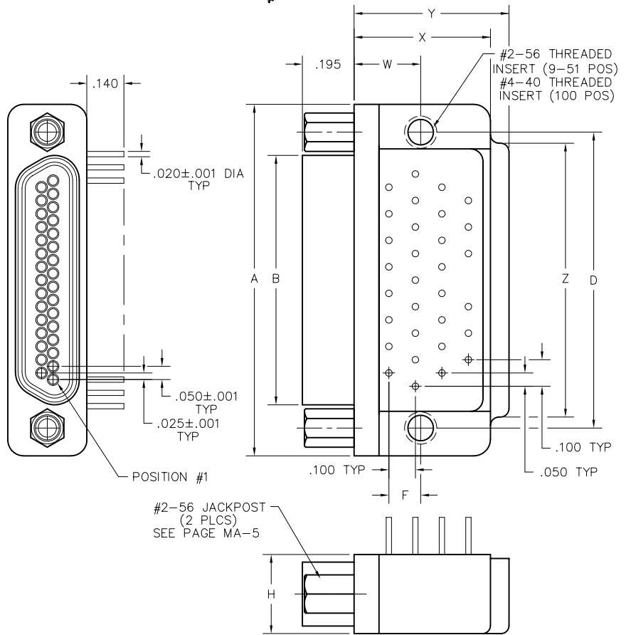
RECEPTACLE
