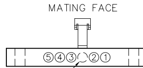
RECEPTACLE MA-121-005-261-A03WA
