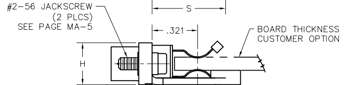
RECEPTACLE
