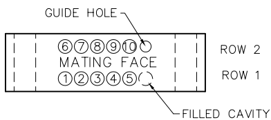
PLUG MA-211-010-161-A66WA
