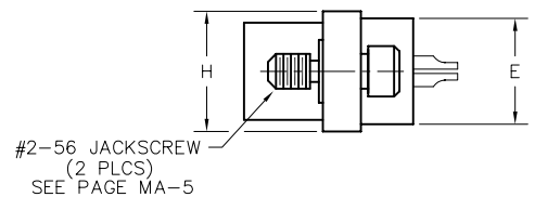
RECEPTACLE
