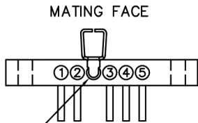
PLUG MA-171-005-325-A0300
