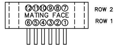
RECEPTACLE MA-281-012-435-A0000
