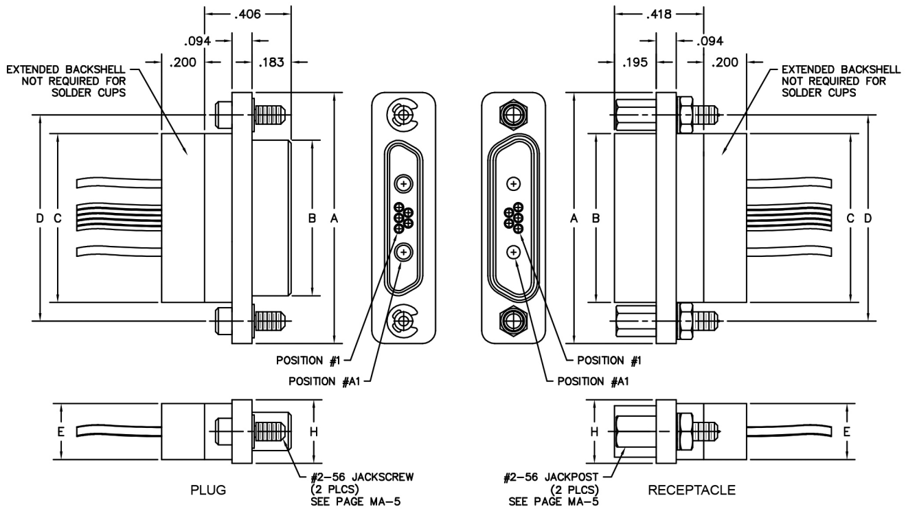
MM-2G2-007-P23-2200 (METAL)
