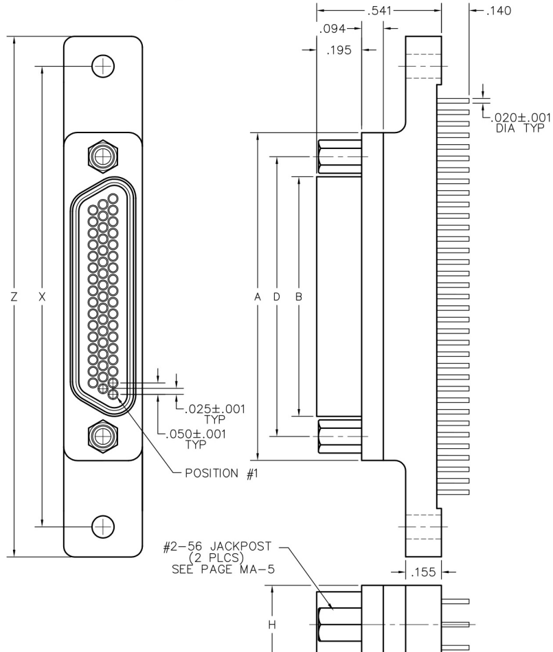
RECEPTACLE
