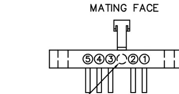
RECEPTACLE MA-181-005-435-A0300
