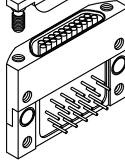
MHT-2E2-021-433-000S (METAL)
