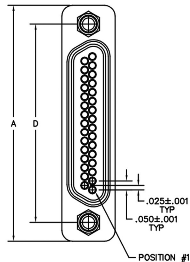
RECEPTACLE
