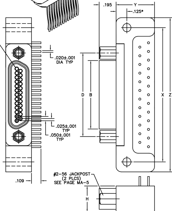
RECEPTACLE
