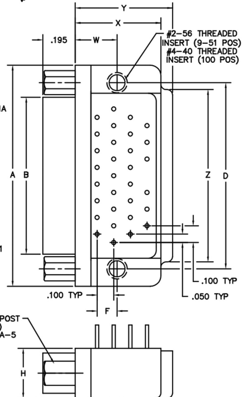
RECEPTACLE
