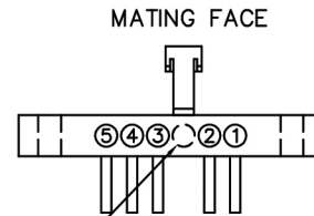
RECEPTACLE MA-181-005-435-A0300
