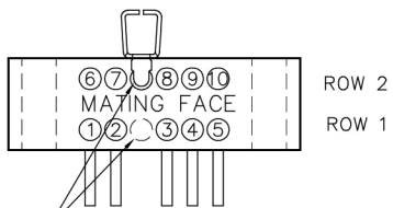
PLUG MA-271-010-325-ABC00
