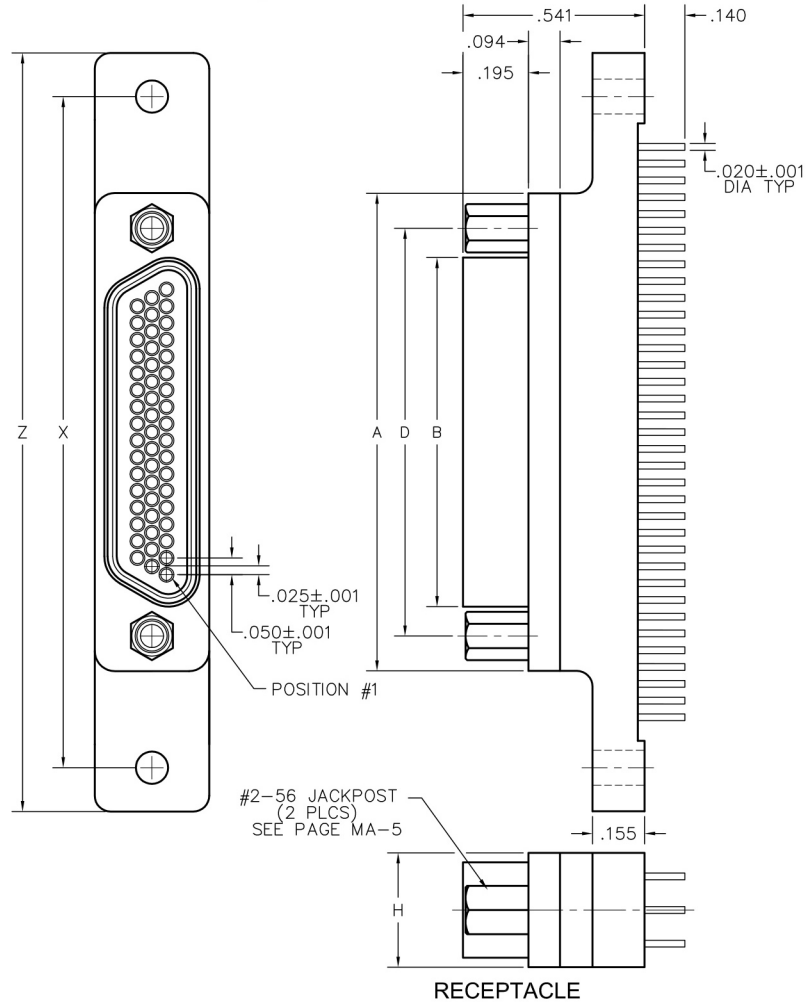
RECEPTACLE
