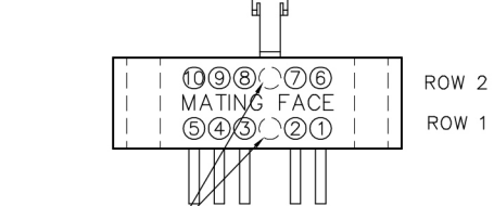
RECEPTACLE MA-281-010-435-ALC00
