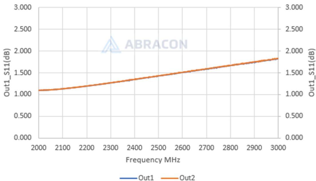
VSWR_S11(2300-2700MHz)
