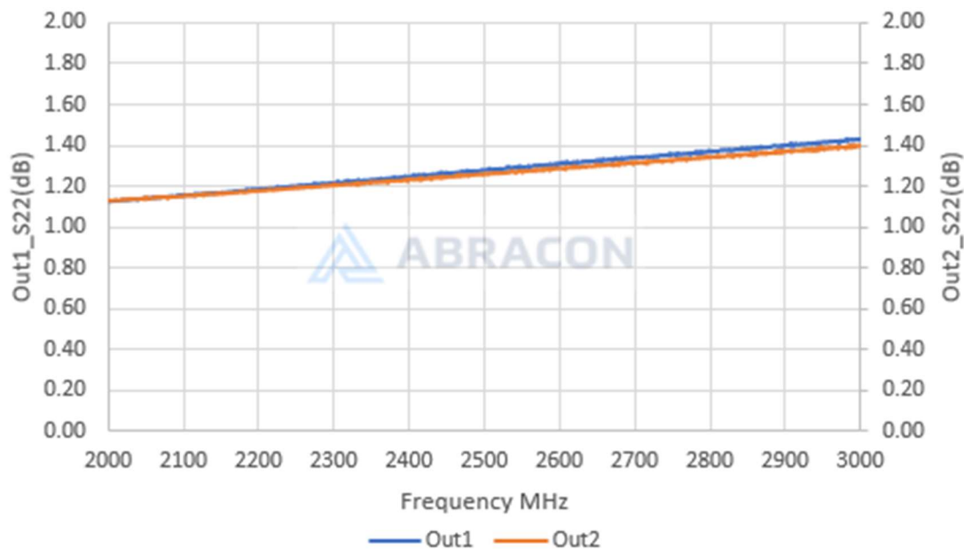
VSWR_S22(2300-2700MHz)
