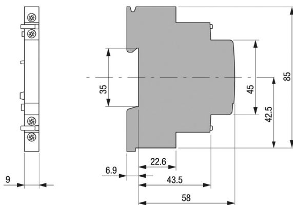
E298 MAIN CONTACT MODULE
