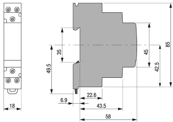
E296-CP COMPENSATOR
