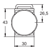
Joystick
