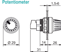
Potentiometer
