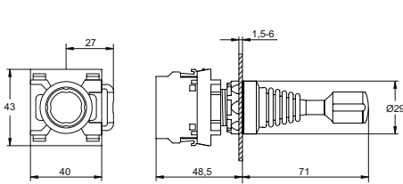
Joystick
