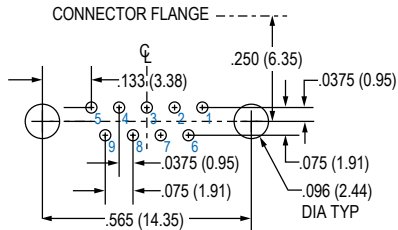
9 SOCKET
