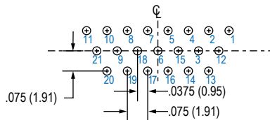
21 SOCKET
