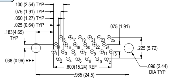
25 SOCKET M83513/31-D
