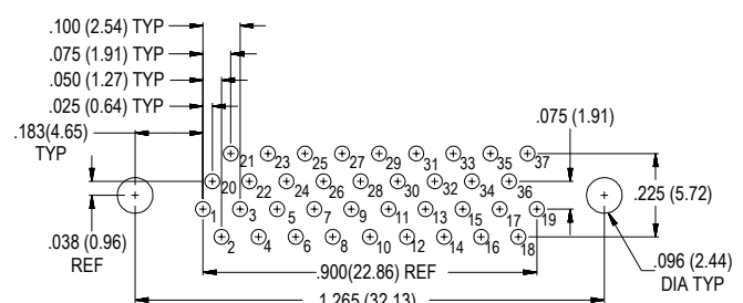
37 SOCKET M83513/31-F
