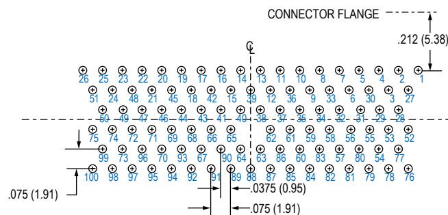
100 SOCKET
