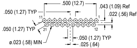
21 Socket
