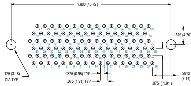
100 SOCKET
