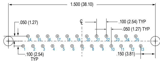
25 SOCKET M83513/25-D
