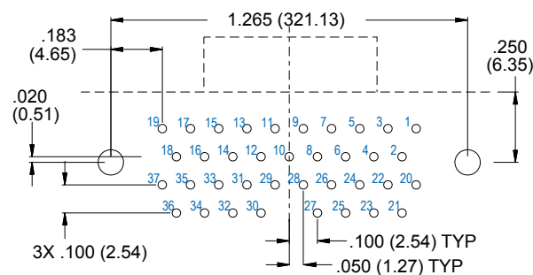
37 Socket
