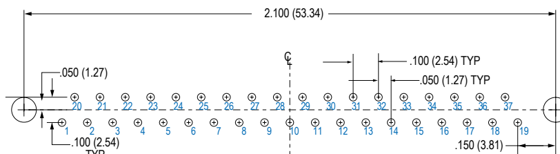
37 SOCKET
