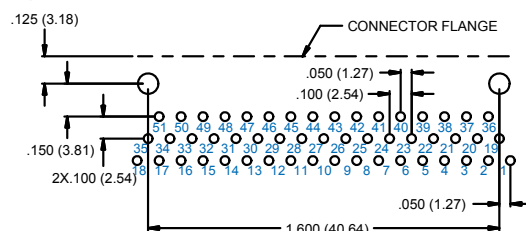
51 PIN M83513/17-G
