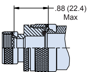
STYLE 2 45° & 90°
