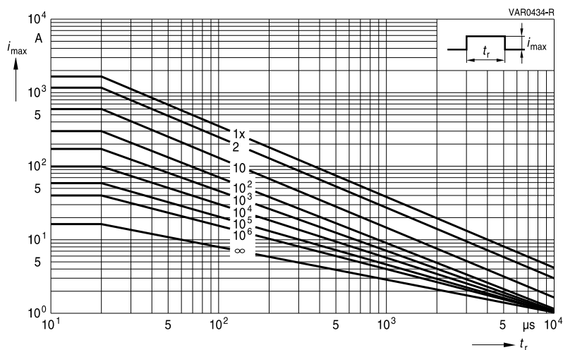
SIOV-S07K130 ... K320E2
