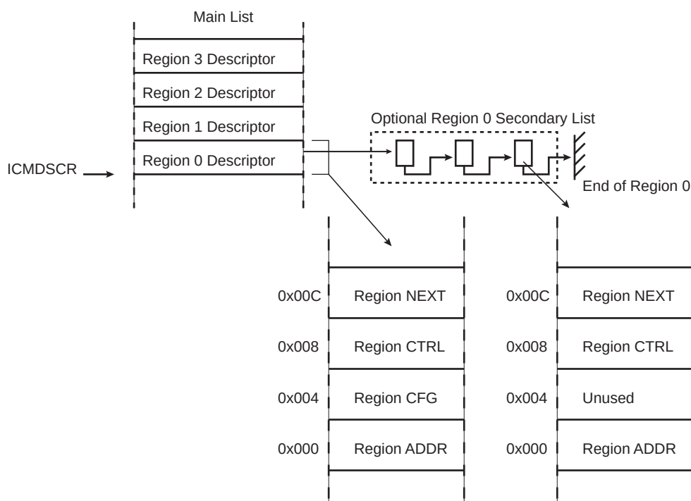
Figure 55-4. Region Descriptor
