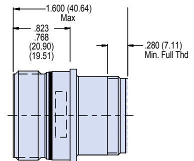
Inline Receptacle
