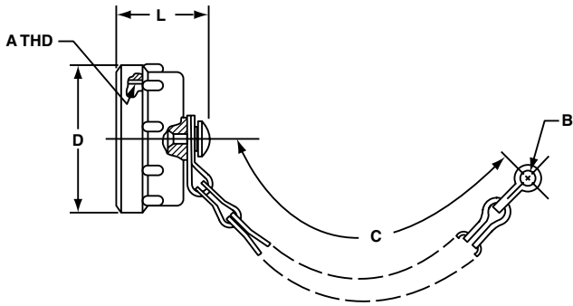
RECEPTACLE PROTECTION CAP 10-422905-
