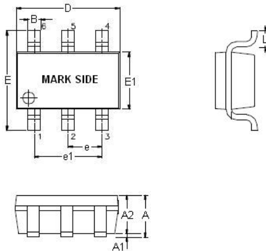
TSOT-23-6 Package (Unit: mm)
