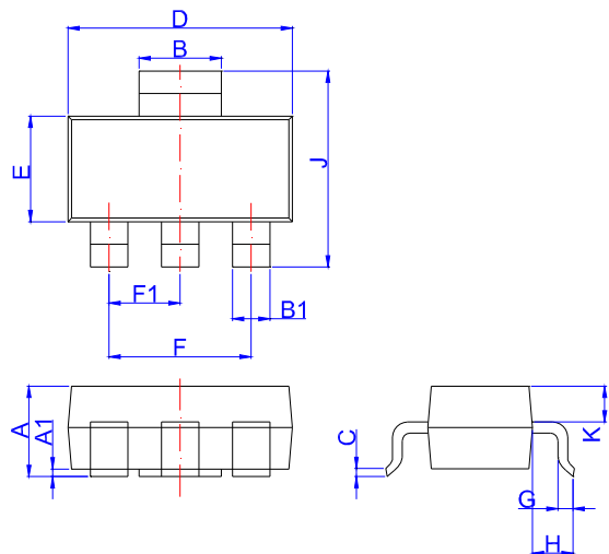
SOT-223
