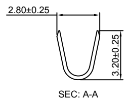
SEC: A-A
