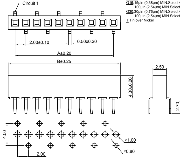
P.C.B LAYOUT
