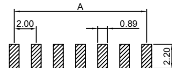
P.C.B LAYOUT
