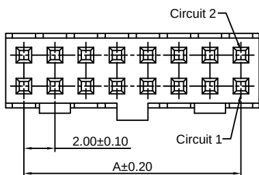
2x2P~2x25P A2005HB-N-2xXP-E
