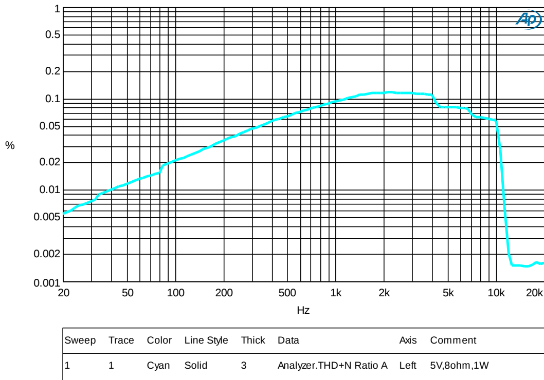
图 6. VDD=5V, R L =8Ω, P O =1W 时的 THD+N
