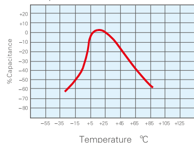
2F4 温度特性曲线 Temperature Coefficient
