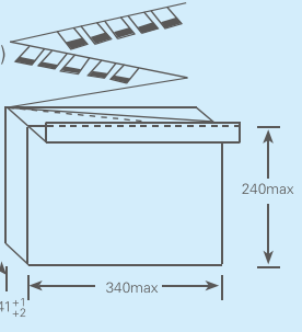
图3 盒装尺寸(mm)
