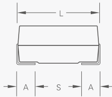
正视图
