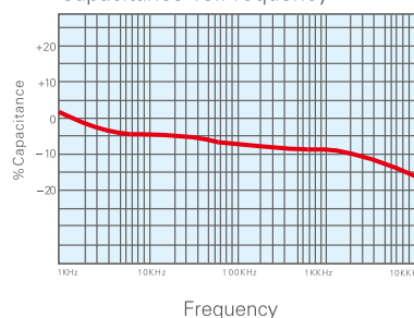
2X1 频率特性曲线 Capacitance vs.Frequency
