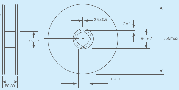
图2 卷装尺寸(mm)
