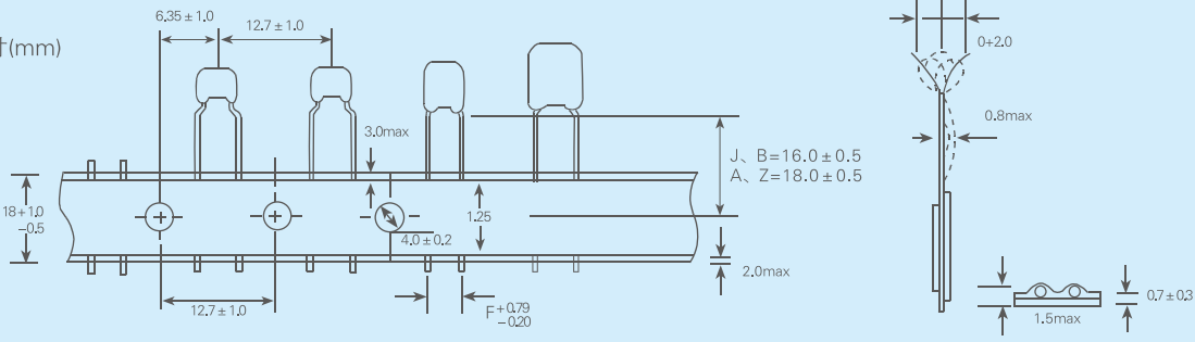
图2 卷装尺寸(mm)
