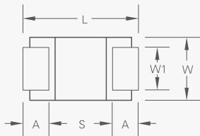
底视图
