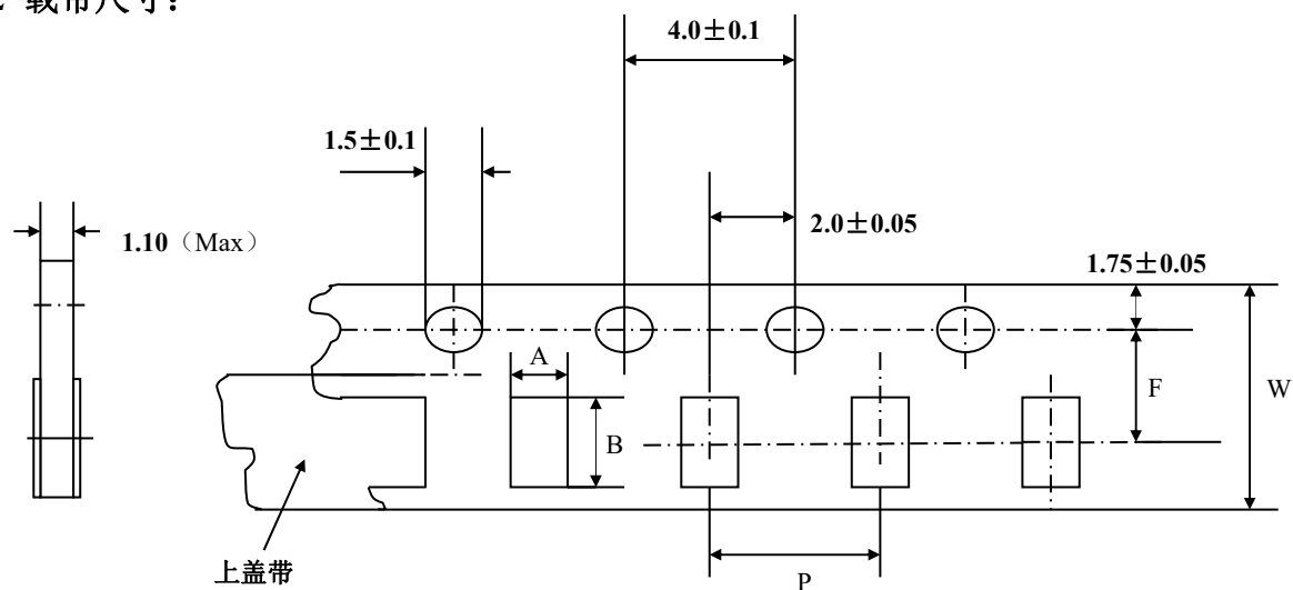
图2 载带
