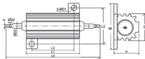
(PDM5 25W~50W)
