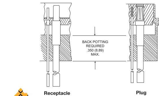
Receptacle
