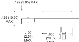
Receptacle
