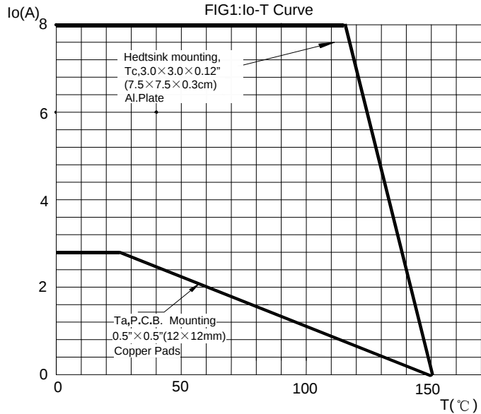
图1: I_o -T 曲线 FIG1: I_o -T Curve
