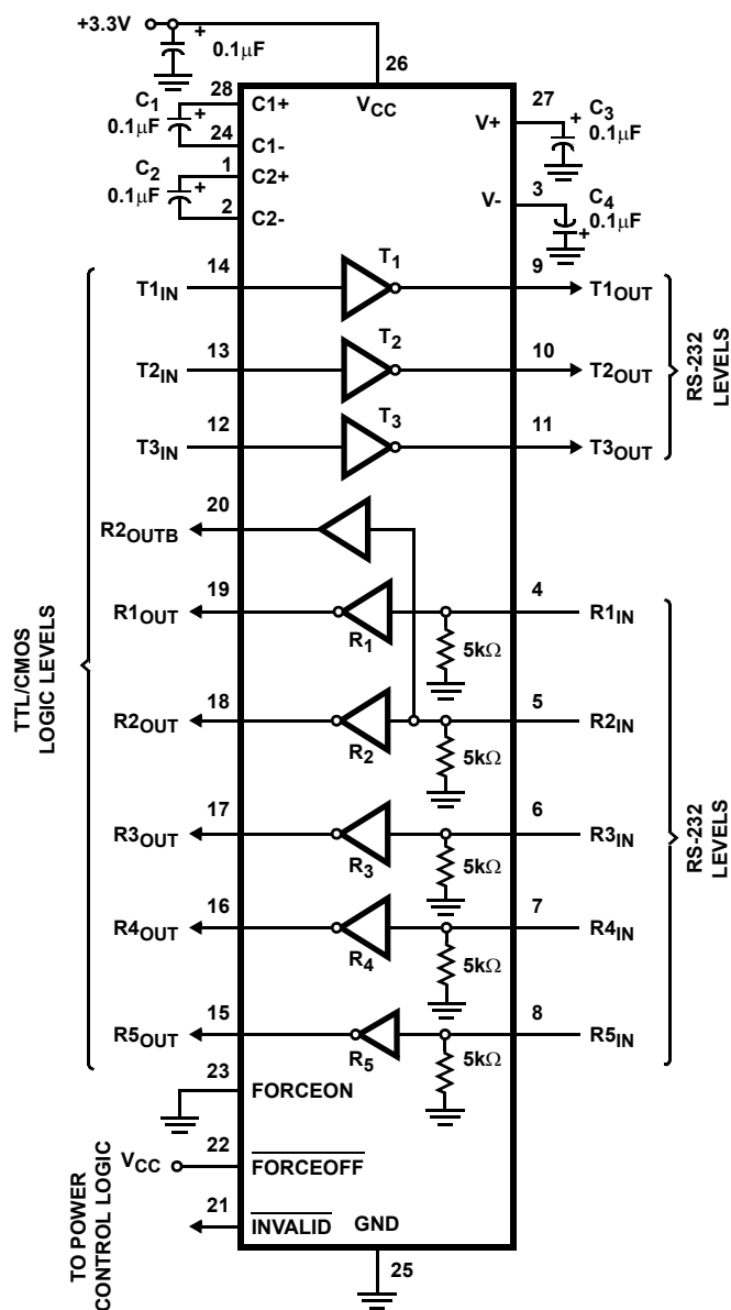
ICL3243
