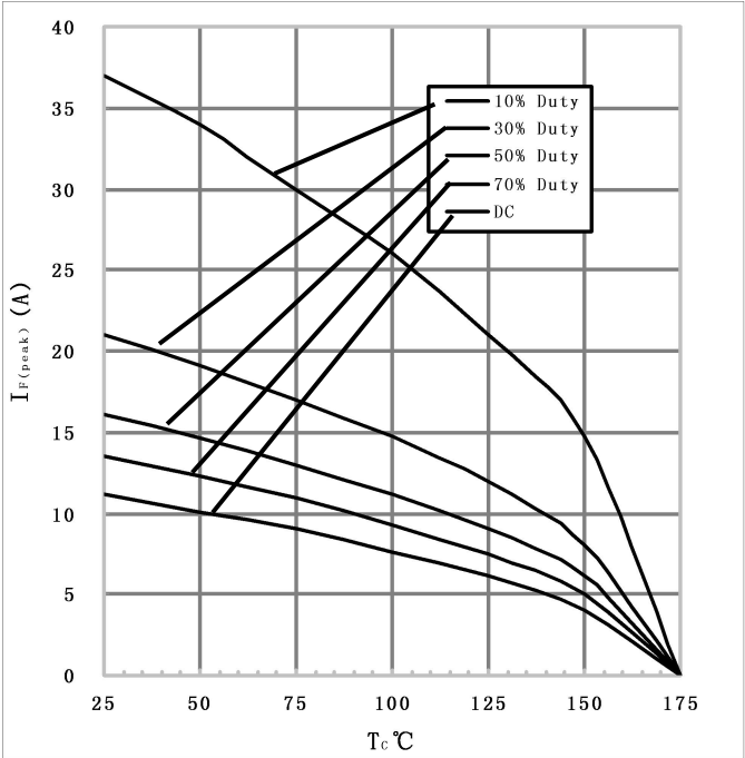
3) 不同负载下的电流（Current Derating） （10%， 30%， 50%， 70%， DC）
