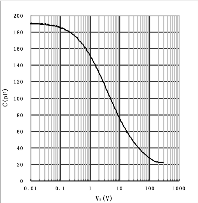
4)典型电容-反向电压曲线
