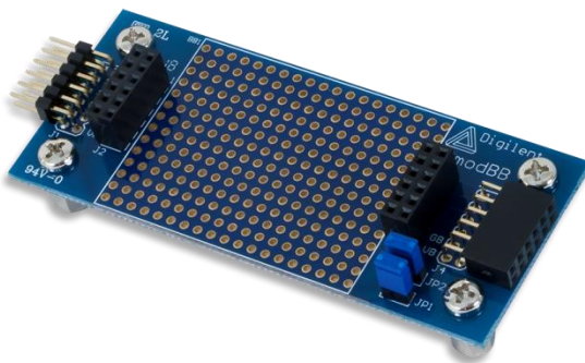
The PmodBB.
